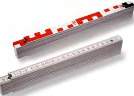
2 m langer Geo-Maßstab – Fernsichtskala mit E-Teilung auf der einen Seite und klassische metrische Skala auf der anderen Seite.
